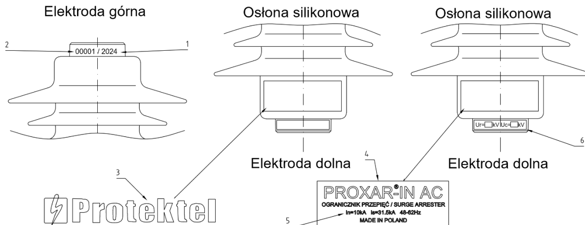
Rys.8. Miejsce cechowania ogranicznika przepięć PROXAR-IN AC
