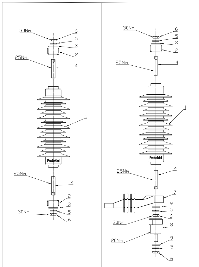
Rys. 6. Ogranicznik przepięć z wspornikiem izolacyjnym i uziomowym i odłącznikiem
